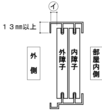
網戸レールと外障子のスキマ ①
