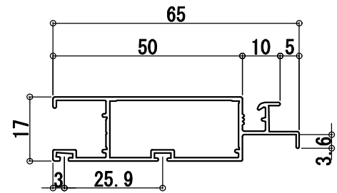
ビル用縦框 1
