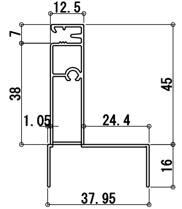
ビル用縦框 1
