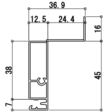
S型上棧
