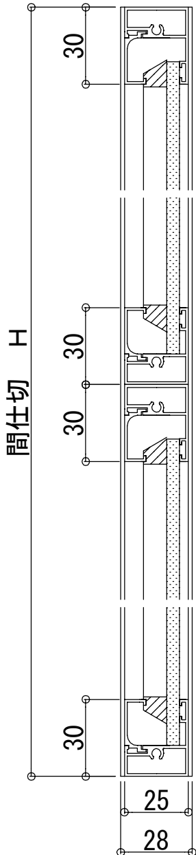
パネル上下枠 (押し縁付)
