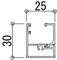
パネル上下枠 (押し縁付)
