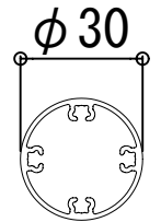
丸束
