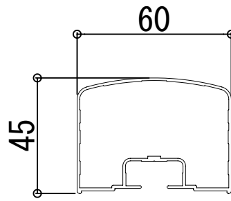
角笠木
