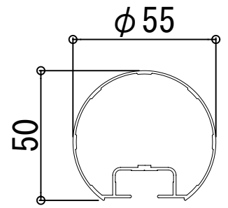
丸笠木
