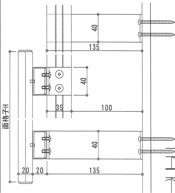
ポール使用壁付け納まり
